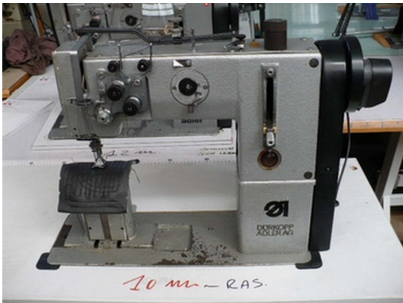
DURKOPP-ADLER 268-FA-273
